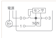
(2線式配線図)
