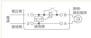
(4線式配線図)
