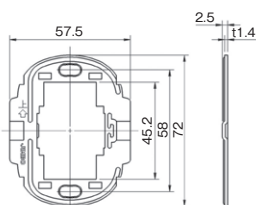
エレガンスミニプレート専用取付枠 1コ用 BS-1M
