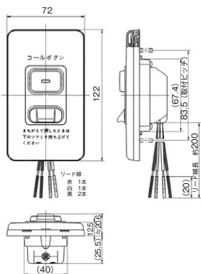
コール用押しボタンスイッチ 解除ボタン付 照光式・自己保持回路内蔵形 HB-70L-DZ
