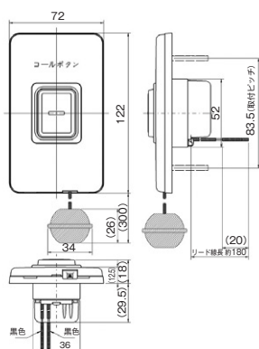
コール用押しボタンスイッチ プルスイッチ付 モーメンタリー形(常開形) HB-80
