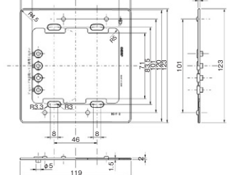
絶縁フレーム 2 連用 BS-F-2
