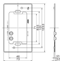
絶縁フレーム 1 連用 BS-F
