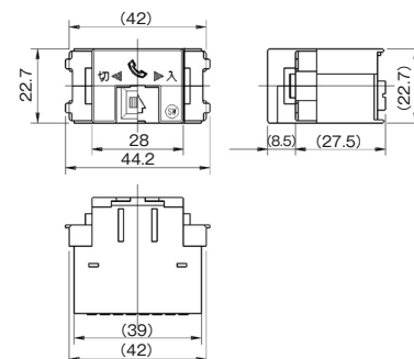
電話用 埋込分離器 JEC-BN-CM6J PW
