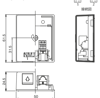
露出形モジュラジャック コンデンサ付 6極2心2口用 NMJ-22CA
