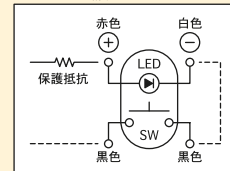
HB-60L 回路図
