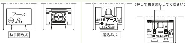
抜止接地ダブル 絶縁枠 JEC-BN-99GV PW
