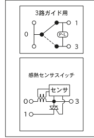
回路図
