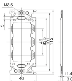
埋込取付枠 金属枠 BS-C
