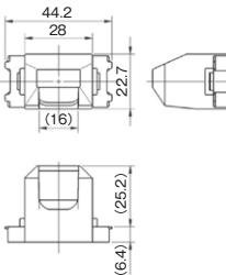
テレホンチップφ16用 JEC-BN-TH PW
