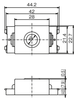
テレホンチップ 丸穴φ9用 JEC-BN-T PW
