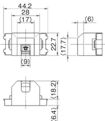
テレホンチップφ9用 JEC-BN-TL PW
