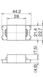
ブランクチップ JEC-BN-0 PW
