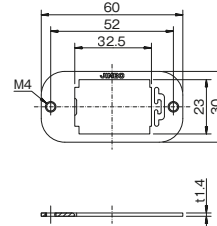
機器用取付枠 BS-A
