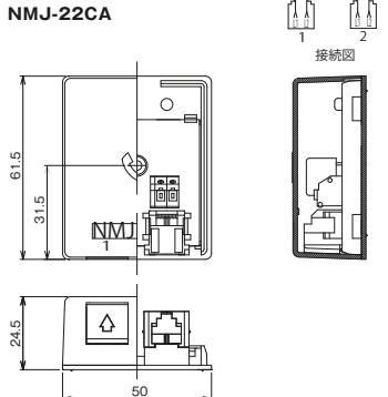
露出形モジュラジャック コンデンサ付 6極2心2口用 NMJ-22CA
