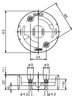
コンセント付 引掛露出ローセットボディ 1384 PW
