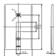
複式コンセントプレート トグルスイッチ用 803A
