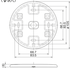
エレガンス丸形blankプレート 丸形 BPN-0UR PW BPN-TUR PW (φ9穴)
