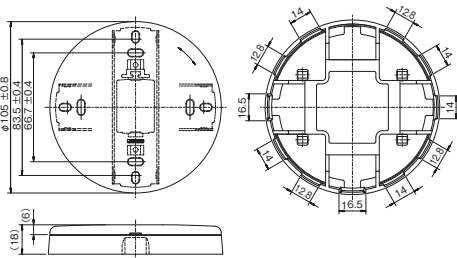
エレガンス丸形blankプレート 丸形 BPN-0UR PW BPN-TUR PW (φ9穴)
