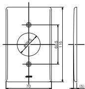
コンセントプレート 1連用 804A
