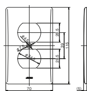
複式コンセントプレート 1連用 807A
