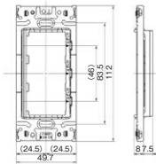
簡易耐火枠 1 連用 WJT-1K
