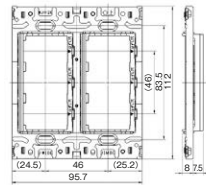
簡易耐火枠 2 連用 WJT-2K
