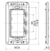
操作板 トリプル マークなし WJN-T1 WJN-T
