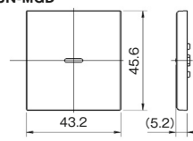
操作板 ダブル マーク付 WJN-GD WJN-MD1 WJN-MD WJN-MGD
