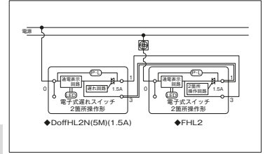
結線図
