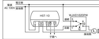
組み合わせ配線図 玄関用 HST-10 の場合
