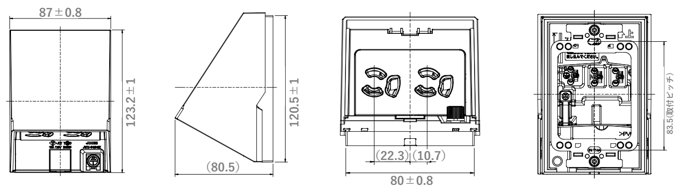
寸法図
