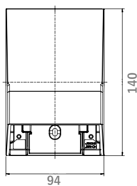
寸法図
