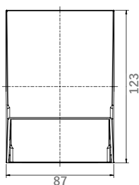
寸法図
