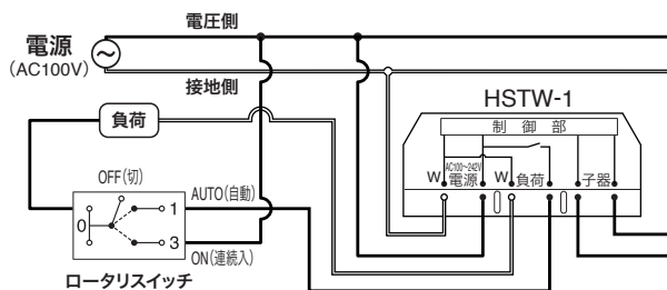
参考配線図(当社HSTW-1との組合せ例)
