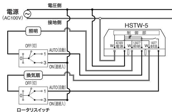
参考配線図 (当社 HSTW-5 との組合せ例)
