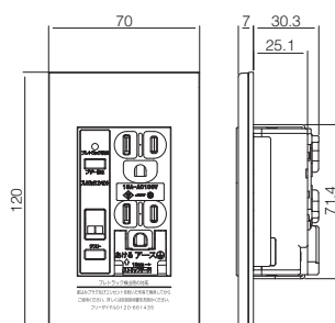
■プレート組合せ寸法図
