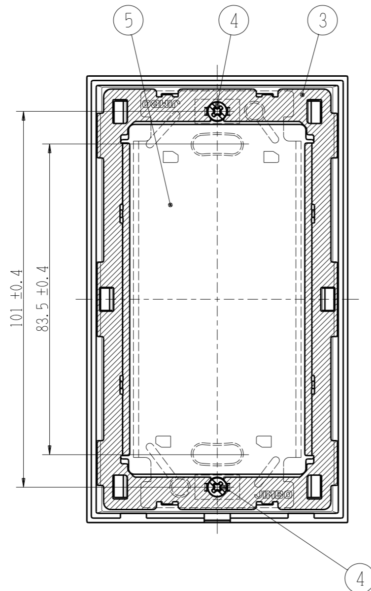
カバープレート未装着図
