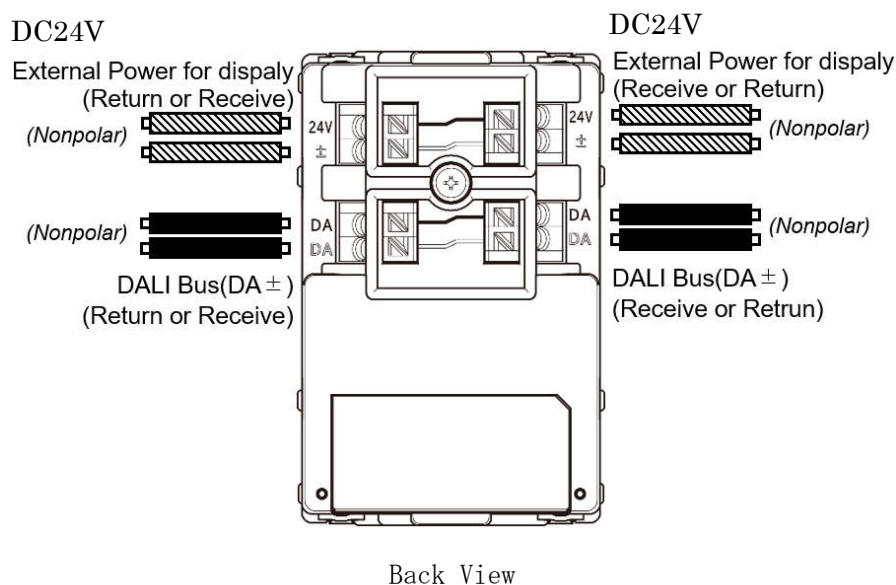
図 2. 配線
