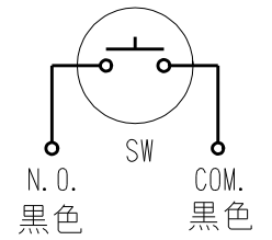
内部結線図
