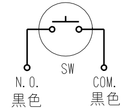
内部結線図
