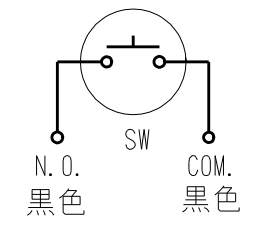
内部結線図
