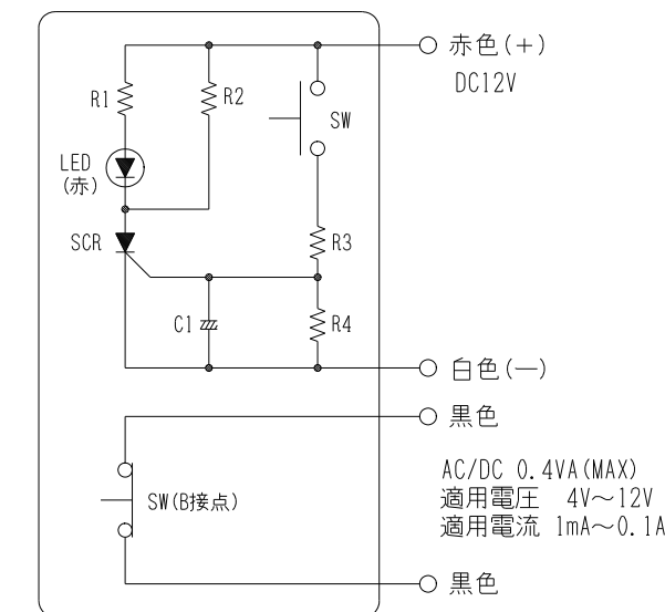
内部回路図
