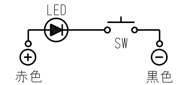
内部結線図
