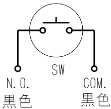
内部結線図
