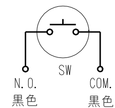
内部結線図
