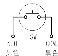
内部結線図
