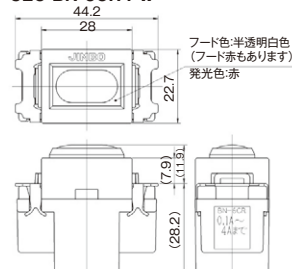
パイロットランプ 電流検知形 4A用 JEC-BN-6CR PW
