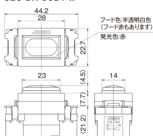
パイロットランプ 電流検知形 0.5A用 JEC-BN-6CL PW
