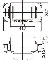
押ボタンスイッチ A接点 JEC-BN-8M PW 押ボタンスイッチ B接点 JEC-BN-8MB PW
