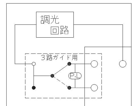
回路図
