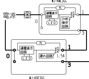
遅れスイッチ配線図
