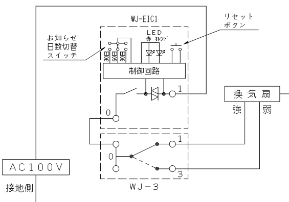
組合せ結線例（下側3路スイッチによる 換気扇 弱強切換）
