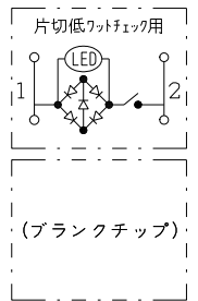
回路図
