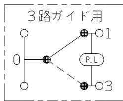
回路図
