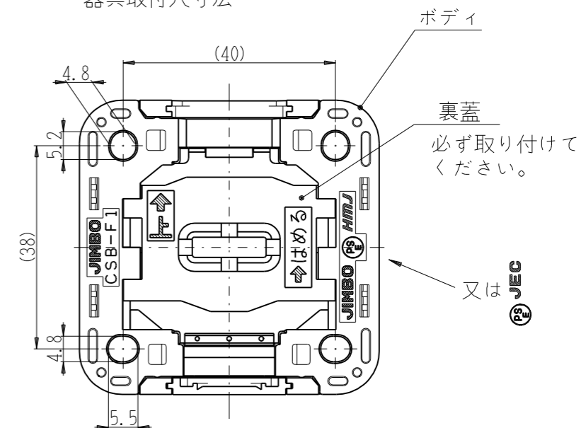
器具取付穴寸法
