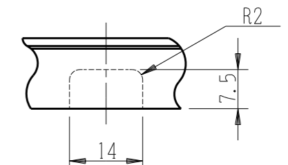
Fケーブル3芯用 引出口-5箇所
