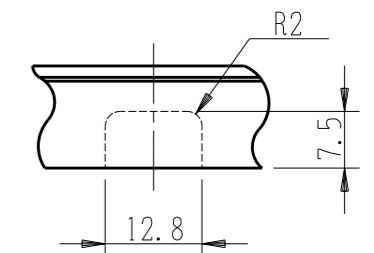
Fケーブル2芯用 引出口-4箇所
