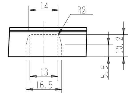
Fモールド1号用 引出口-2箇所
